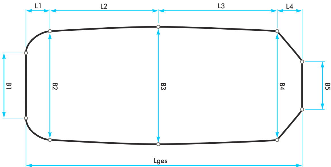
Ansicht seitlich
